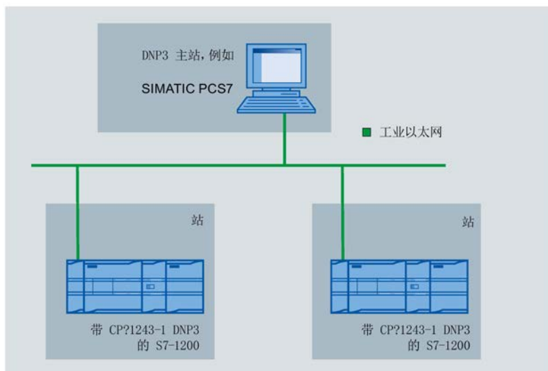
图 1-1 采用非冗余控制中心并且从站处于同一 IP 子网中的组态示例
