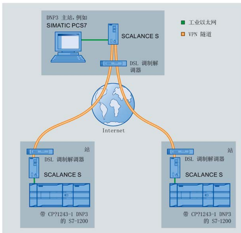
图 1-2 通过 Internet 进行连接的组态示例
