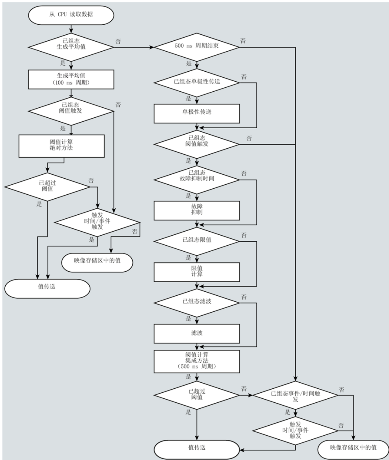
图 5-2 模拟值预处理的顺序
