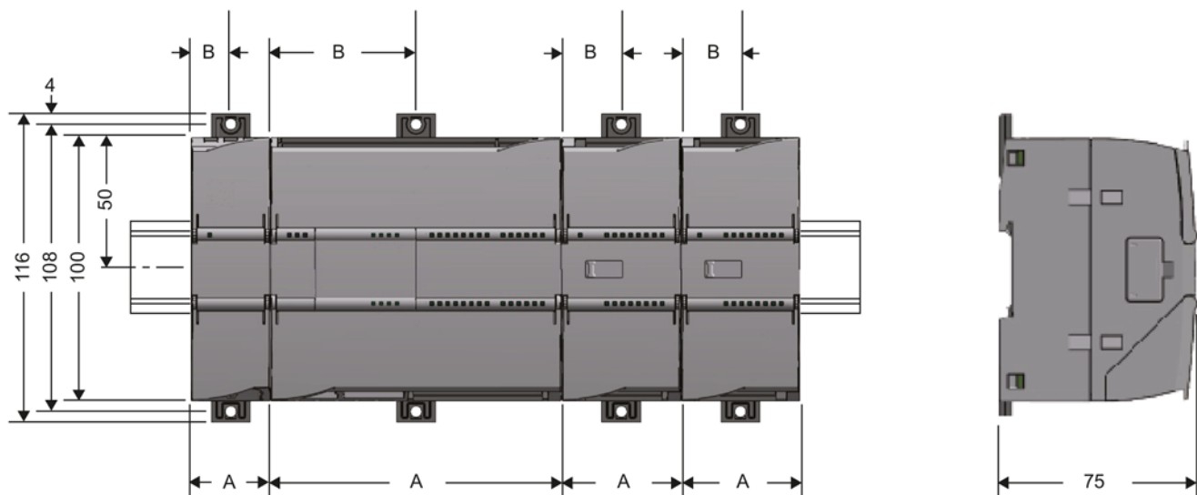
图 4-1 S7-1200 的安装尺寸
