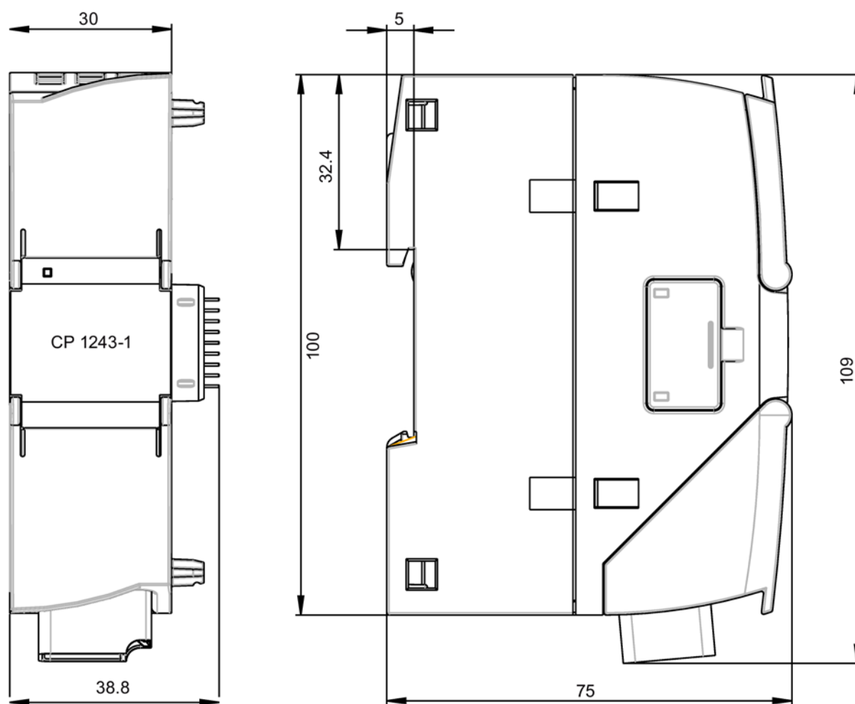
图 B-1 CP 1243-1 DNP3 / CP 1243-1 IEC: 正视图与左侧视图
