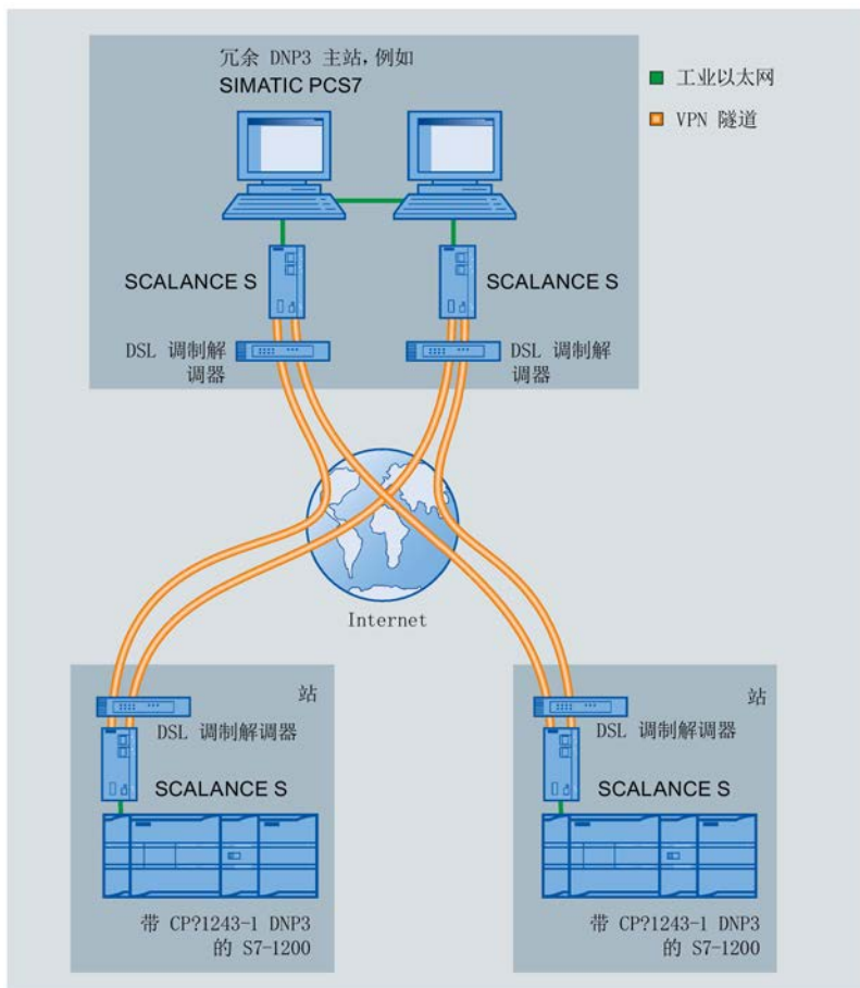
图 1-3 采用冗余 DNP3 主站的组态示例
